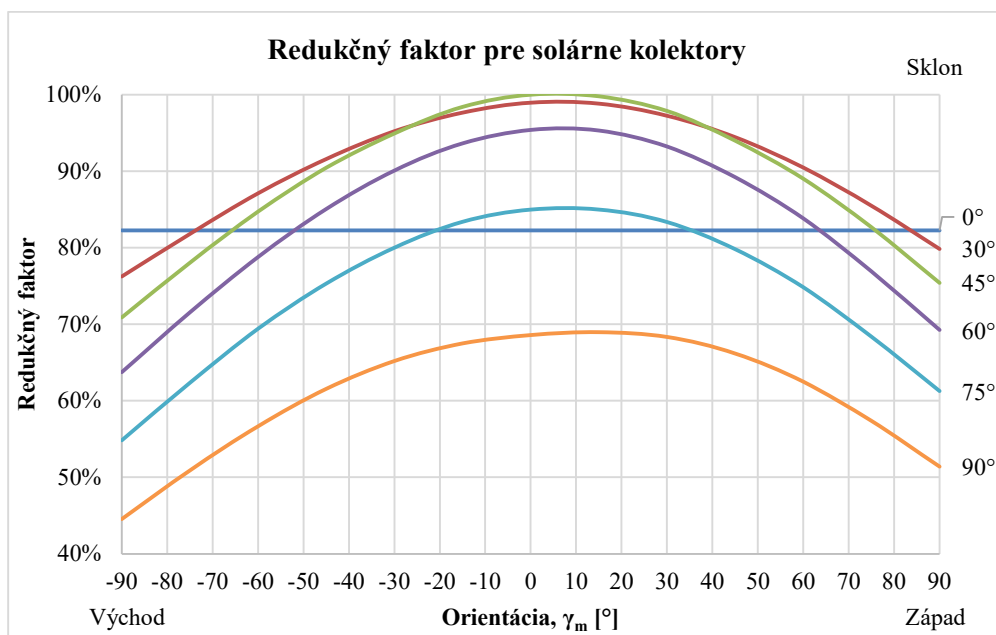
Obr 1. Redukčný faktor (k) pre solárne kolektory
