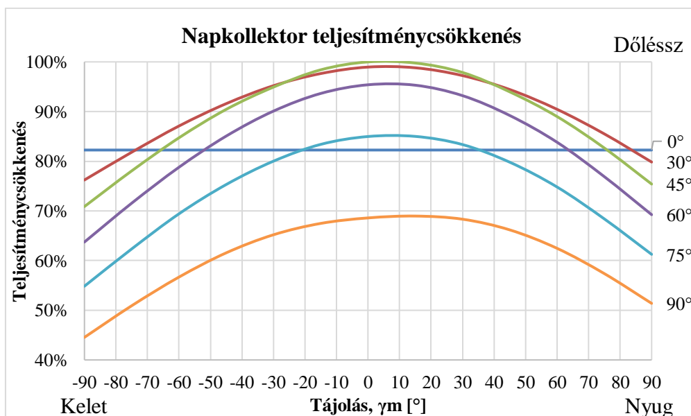
1. ábra, Teljesítménycsökkentő tényező (k) a tájolás és dőlésszög függvényében
